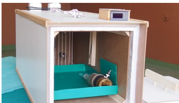
Slika 6. Kutija za prijenos umjetnih vagina s ugrađenim grijačem i termostatom
