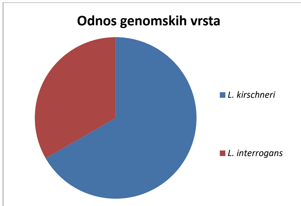
Slika 17. Odnos genomskih vrsta izolata pretraženih u ovom istraživanju pomoću filogenijske analize 245 bp secY gena.
