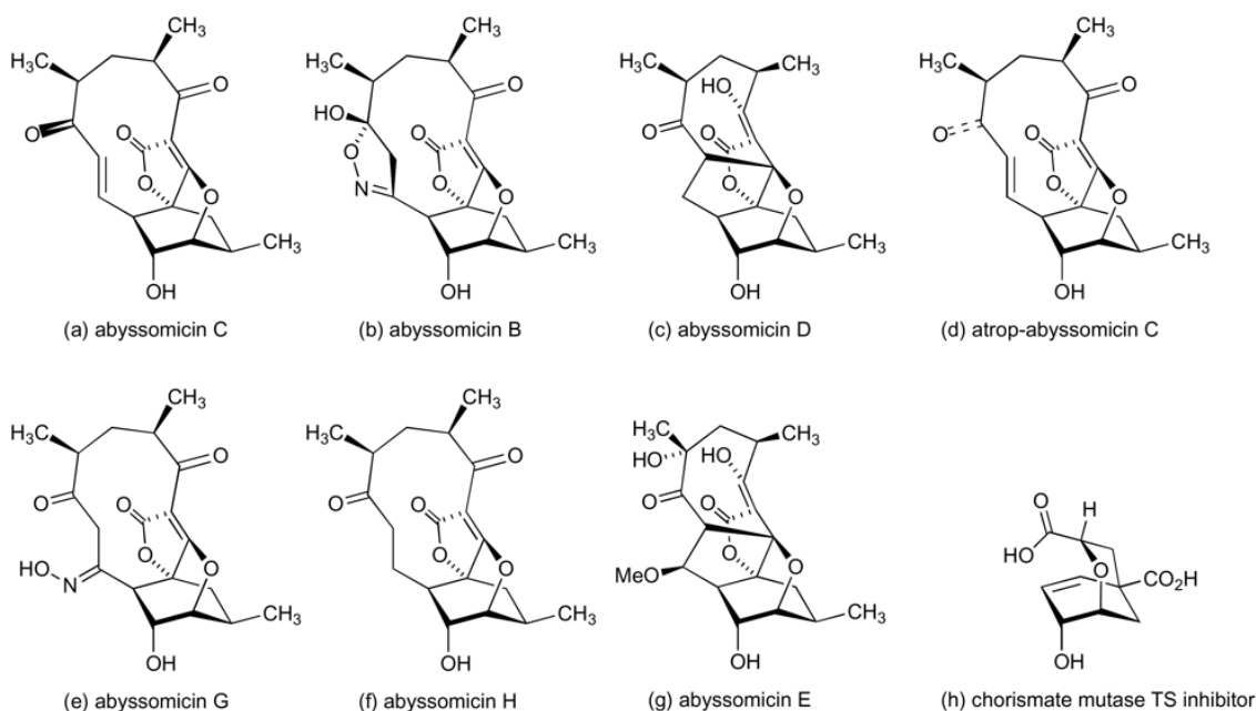
Slika 8. Strukture abisomicina
