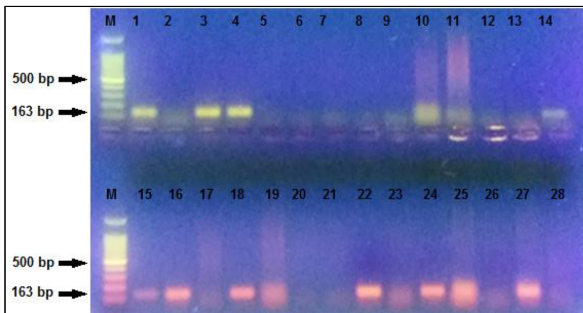
Slika 3. Vizualizacija PCR produkta veličine 163 bp na 1,5 % agaroznom gelu (M- marker; 1, 3, 4, 14, 15, 16, 18, 22, 24, 27 - pozitivni uzorci)
