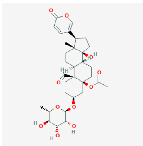
Slika 15 Kemijska struktura lanceotoksina B
