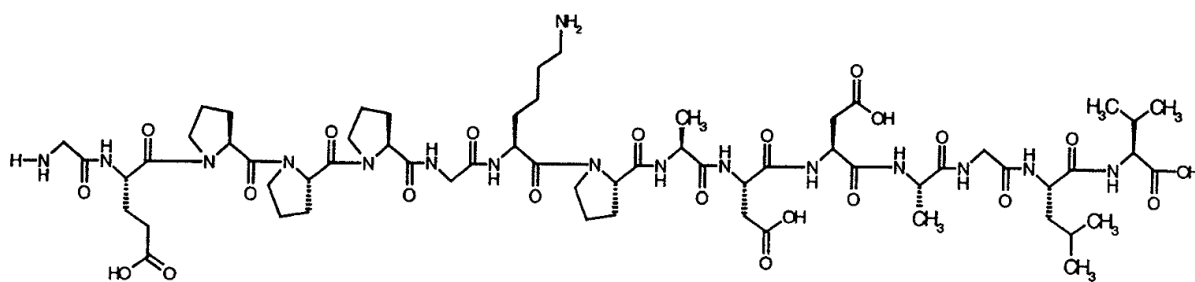
Slika 2. Pentadekapeptid BPC 157
