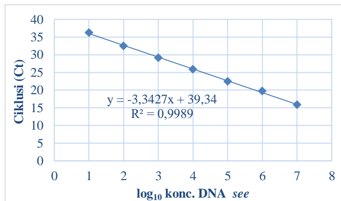
Slika 32. Krivulje amplifikacije i standardna krivulja Real-time PCR reakcije za gen see
